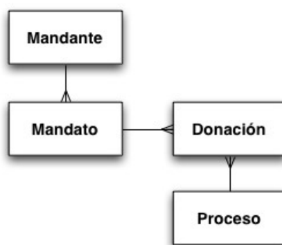
Figura 8: Modelo de clases de la aplicación central
